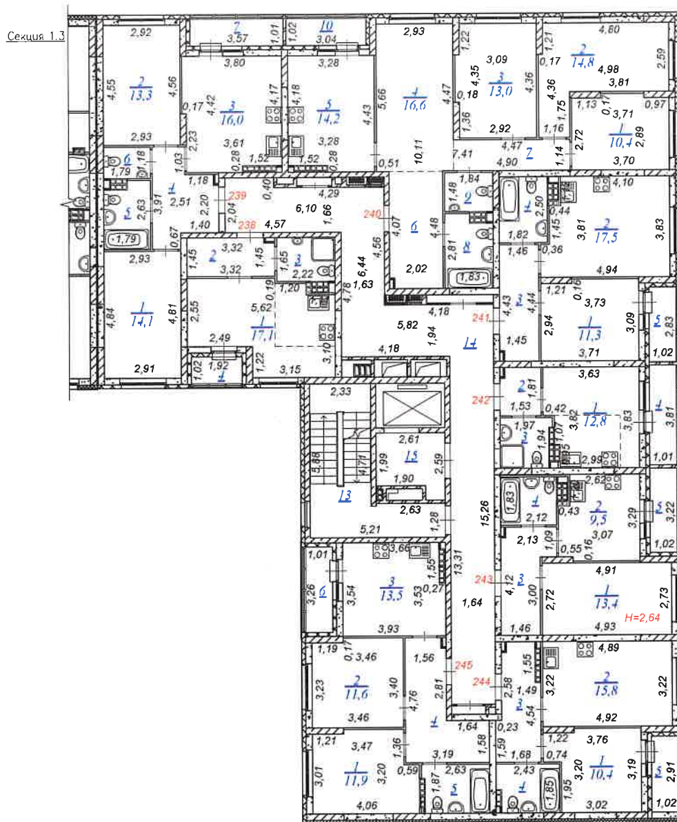
Блокировочная схема
