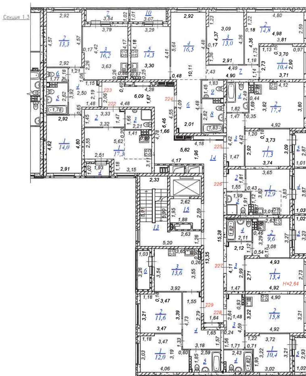
Блокировочная схема
